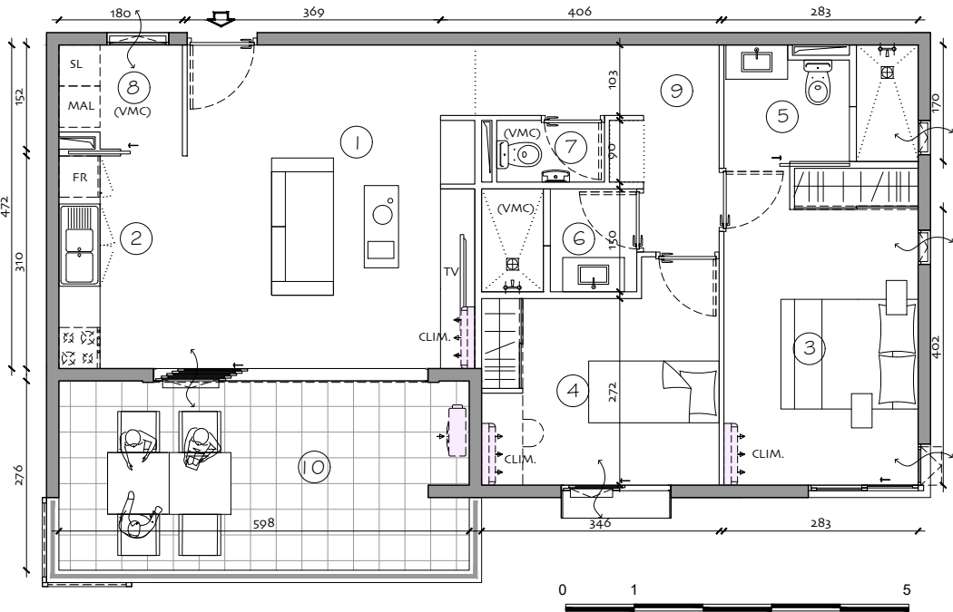
VUE EN PLAN Ech:1/100
