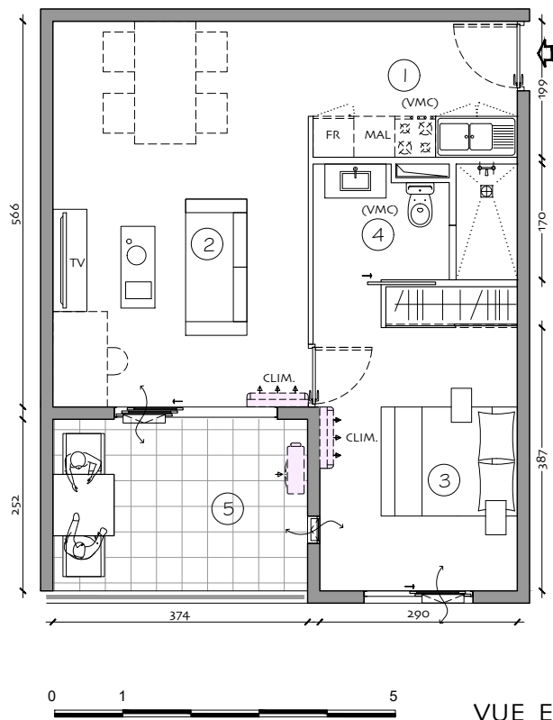
VUE EN PLAN Ech:1/100
