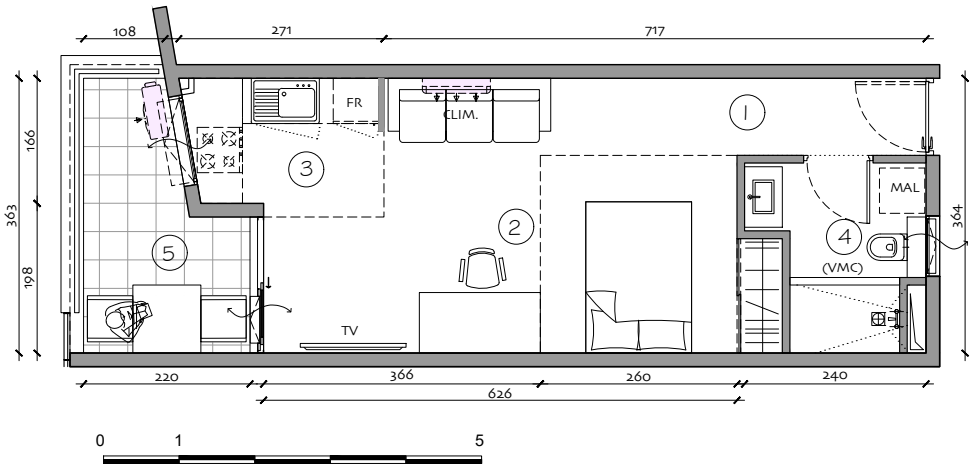
VUE EN PLAN Ech:1/100
